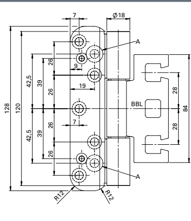
Maßzeichnung Standard / (TZ)
