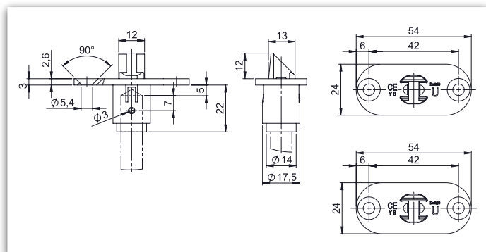
Bemaßung: Schnapsverschluss
