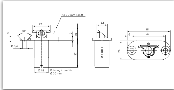
Bemaßung: Schaltverschluss
