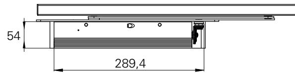
Bemaßung: ECO ITS-630 (3-6)
