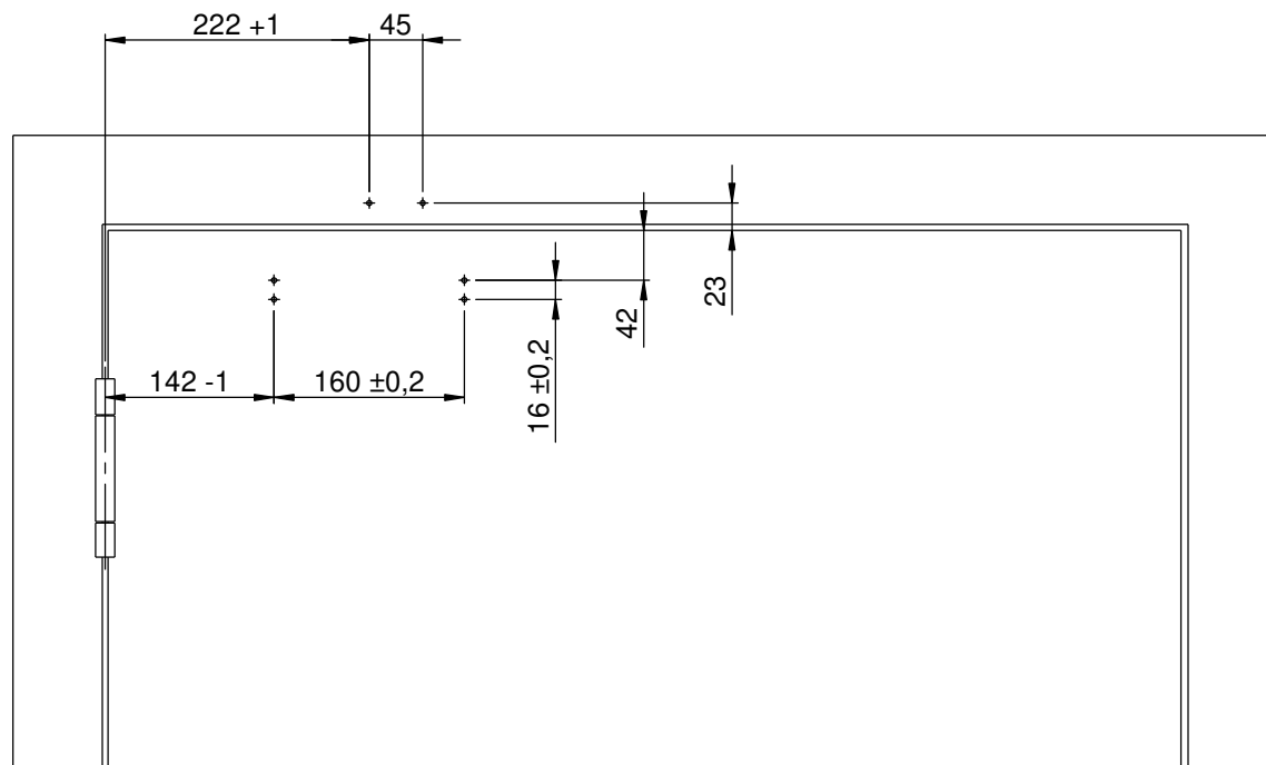
Anbauvariante Direktmontage mit Montageplatte
