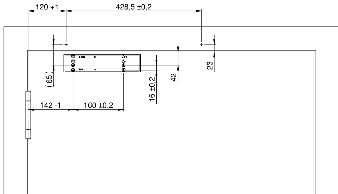
Anbauvariante Direktmontage und Montageplatte
