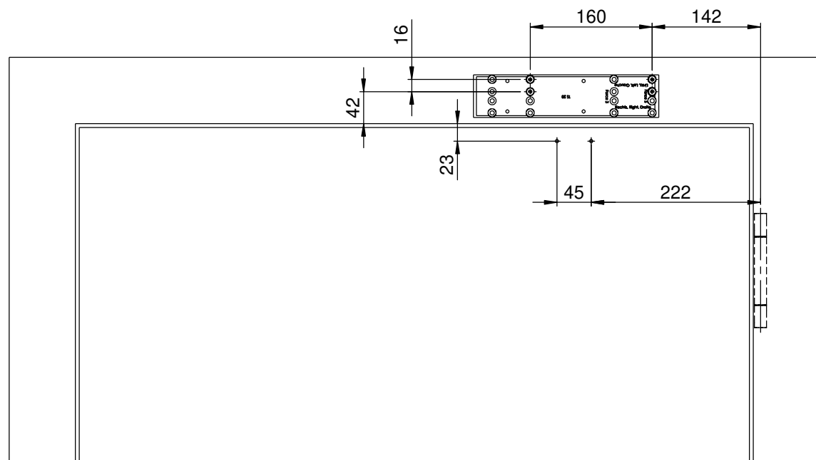
Anbauvariante Montageplatte EN 5
