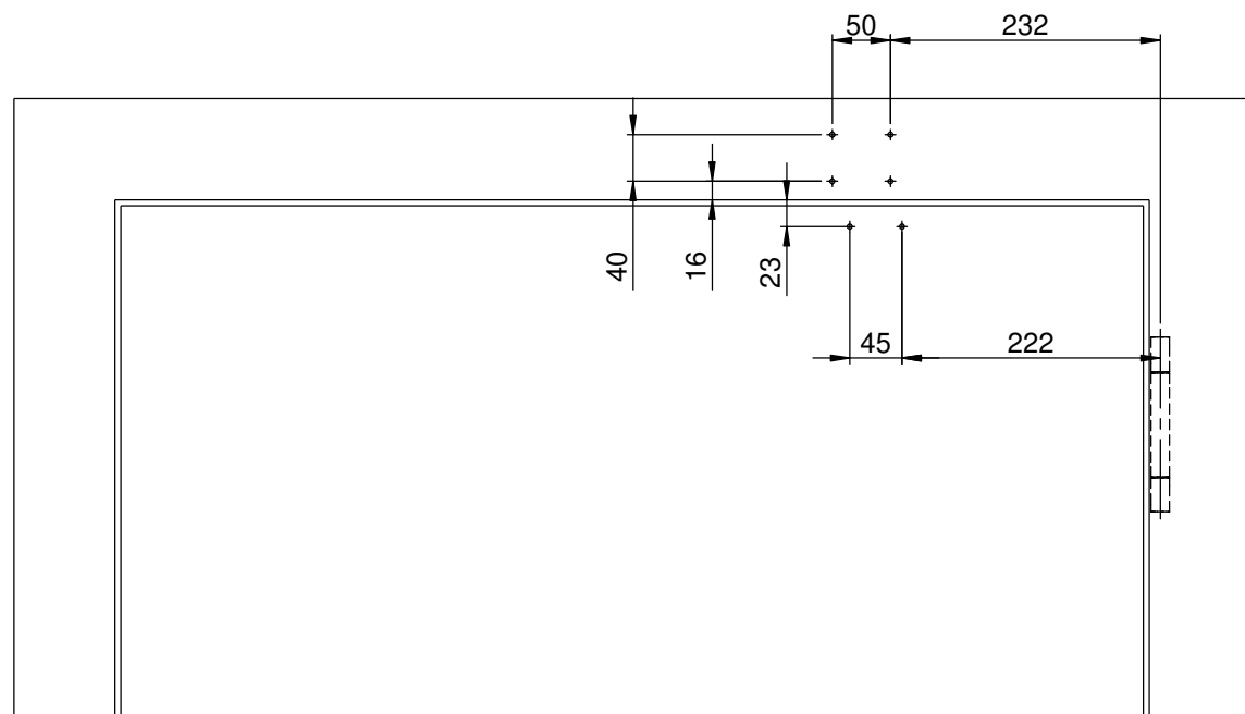
Anbauvariante Direktmontage EN 5
